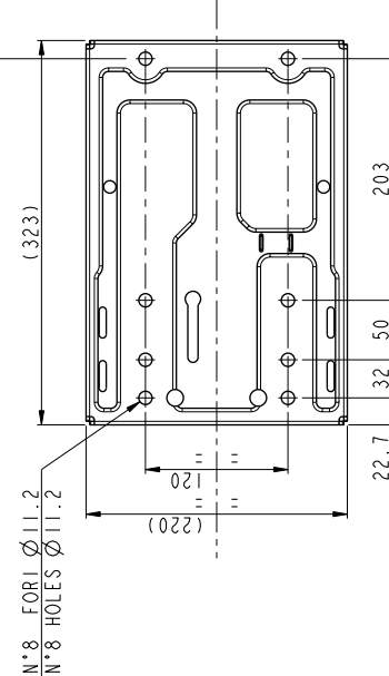
PIASTRA DI FISSAGGIO VISTA DA SOTTO BOTTOM VIEW BASEPLATE
