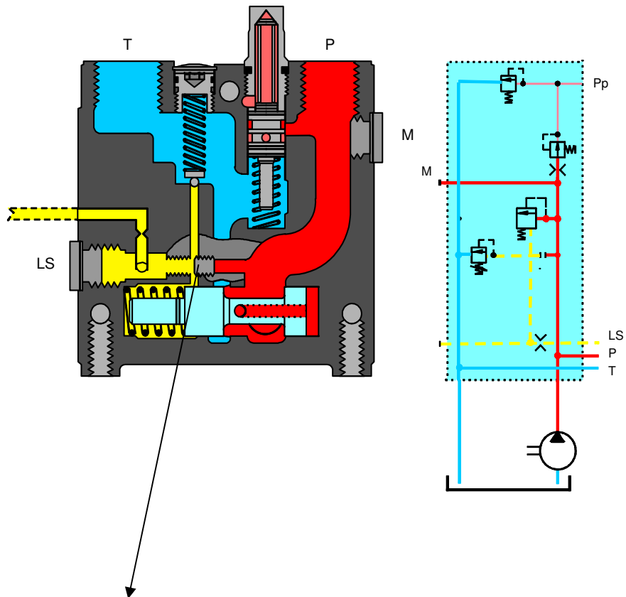
Open Center ( tandwielpompe )
